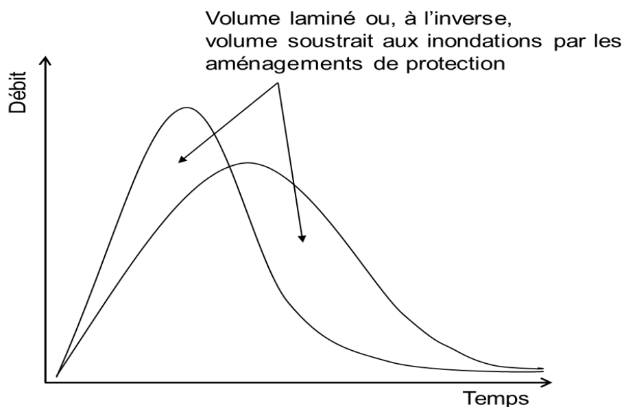
Graphique 2. Le principe de laminage (et son inverse)
