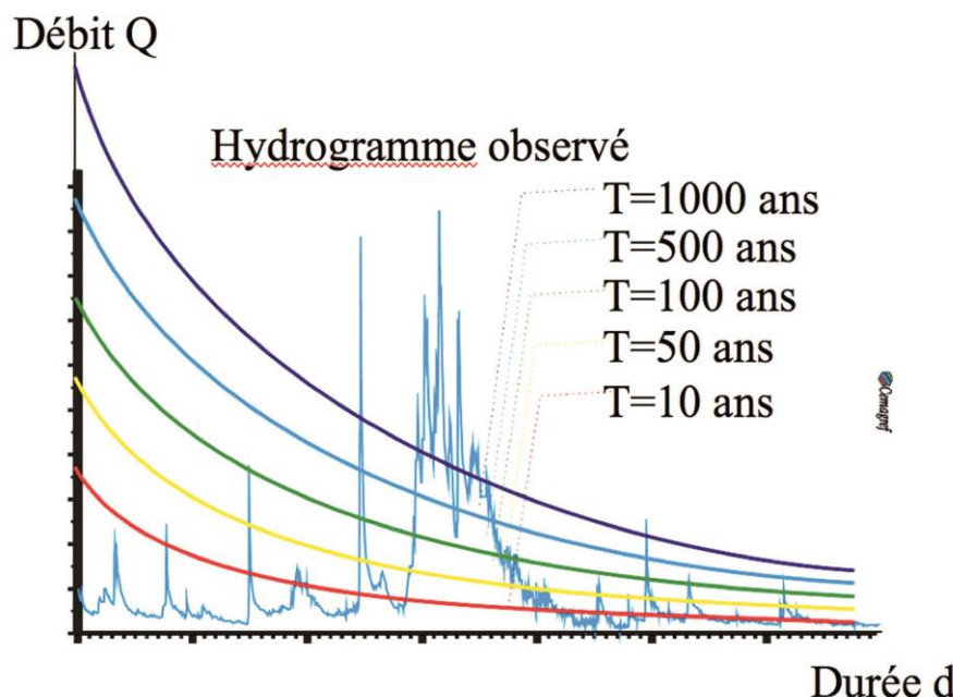
Graphique 1. Les courbes Débit-durée-fréquence (QdF) : Représentation synthétique de l'aléa de crue prenant en compte l'intégralité du régime des crues d'une rivière
