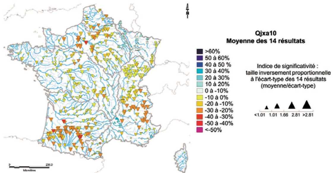
Carte 2. Influence du changement climatique sur les crues des bassins versants français
